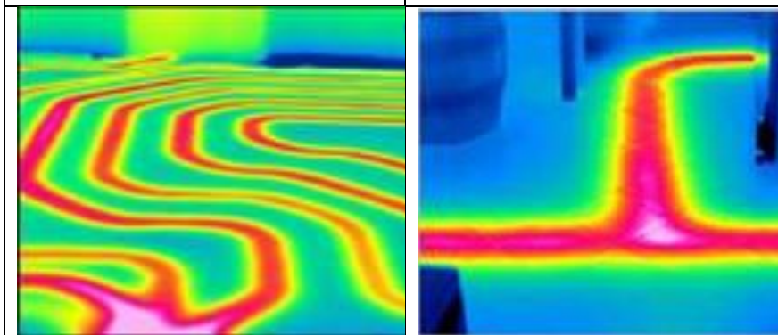
Fot. 10 (na lewo) Przebieg ogrzewania podłogowego Fot. 11 (na prawo) Lokalizacja przebiegu rurociągów grzewczych
