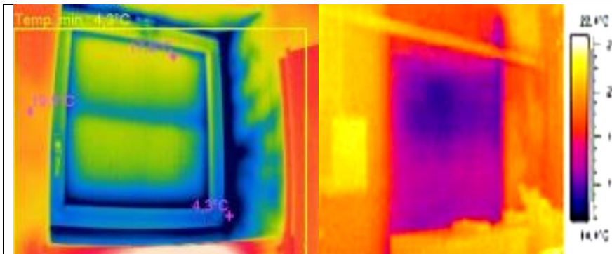
Fot. 8÷9 Termogramy wykonane od wewnątrz - nieprawidłowo osadzone okno (na lewo) oraz zamurwane drzwi (na prawo)
