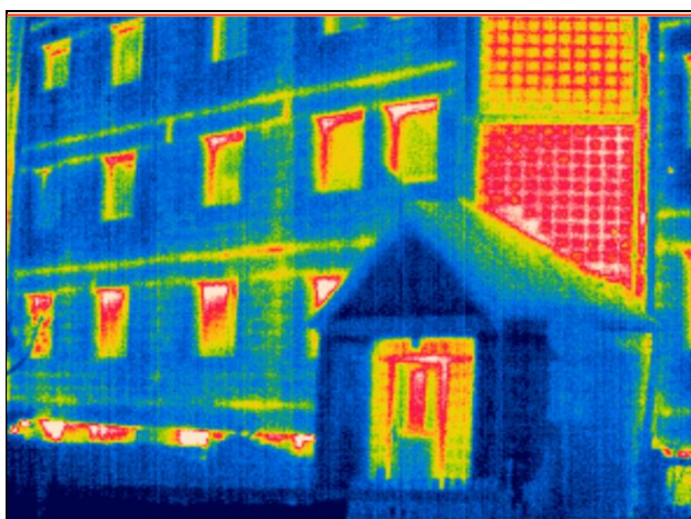
Fot. 5÷6 Zwiększona ucieczka ciepła z budynku przez pustaki szklane (luksfery) stanowiące przeszklenie klatki schodowej
